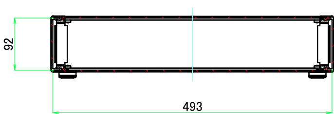
A-A ( 1 : 6.5 )
